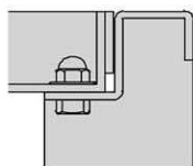
ボルト固定部詳細図
