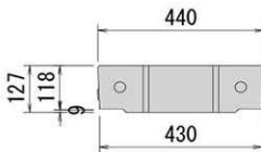
正面図
