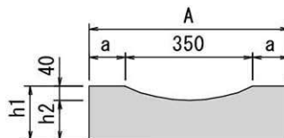
正面图
