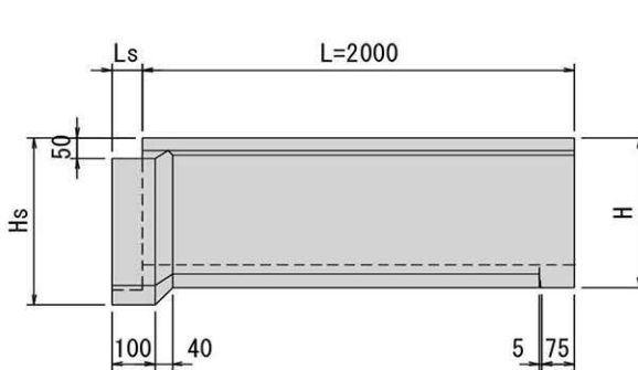
側面図
