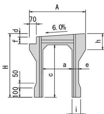
正面図
