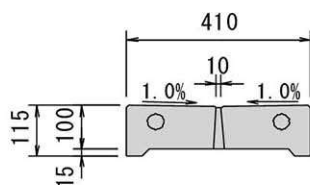
正面図
