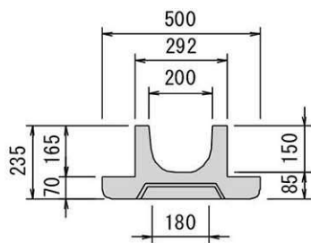
正面図
