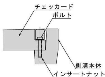
A部（固定部）詳細図
