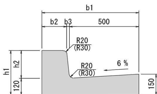
正面図
