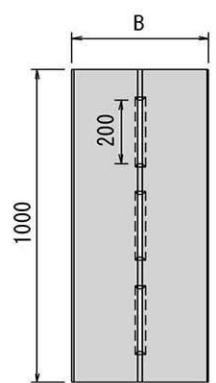
平面図
