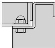
ボルト固定部詳細図
