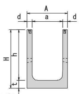
正面図
