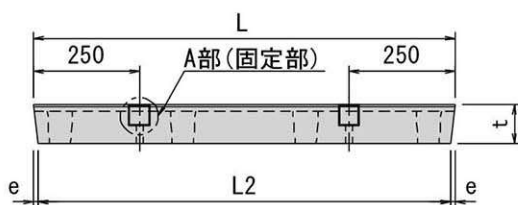
KT側溝・道路側溝（3種）側面図
