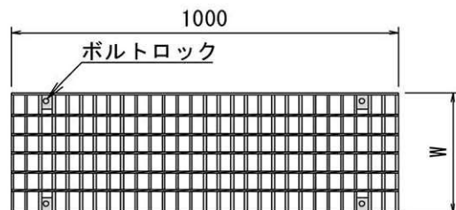
グレーチング平面図
