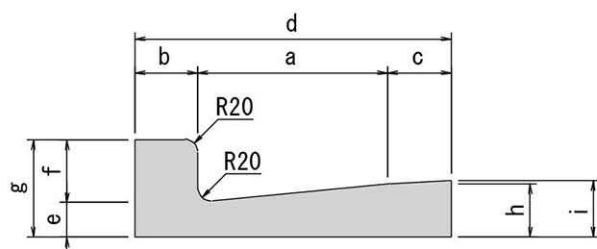
正面図
