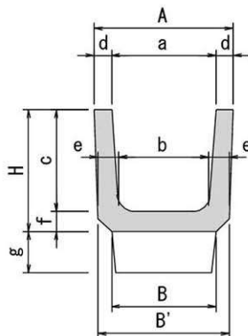
正面図(基本部)
