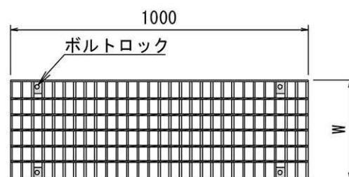
ボルト固定部詳細図
