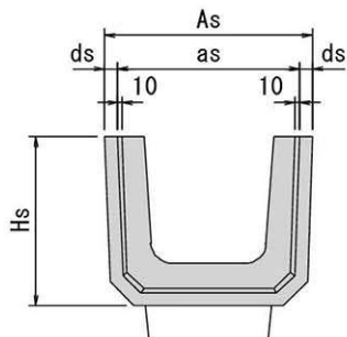
正面図(ソケット部)
