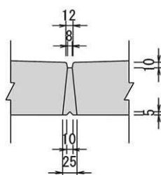
B部（梁部）詳細図
