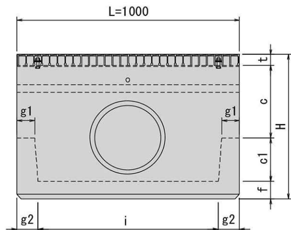
側面図
