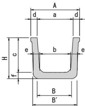
正面図(基本部)
