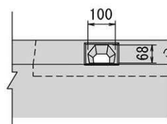
A部 側面図
