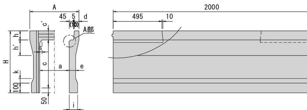
正面図
