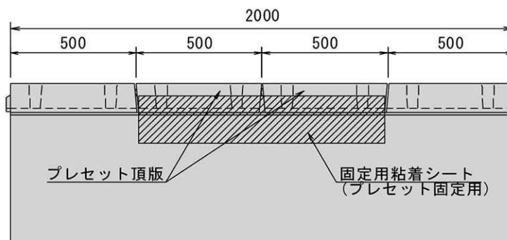
側面図
