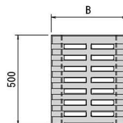
正面図
