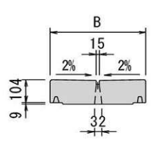
断面図
