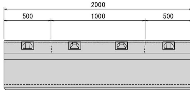
側面図
