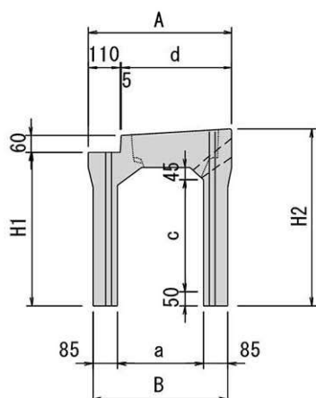
正面図
