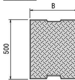
正面図
