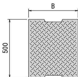
正面図
