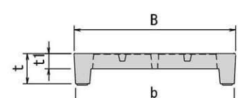
正面図
