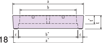
正面図 D
