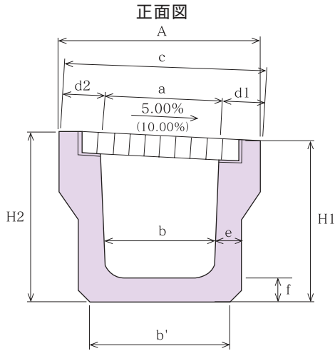
寸法表
