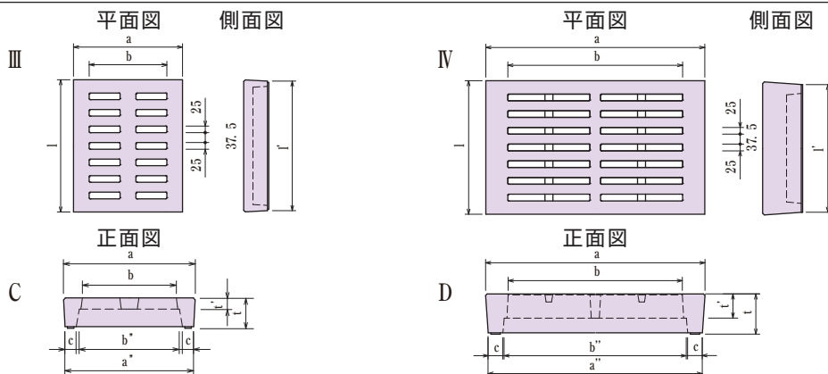
寸法表
