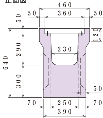
正面図
