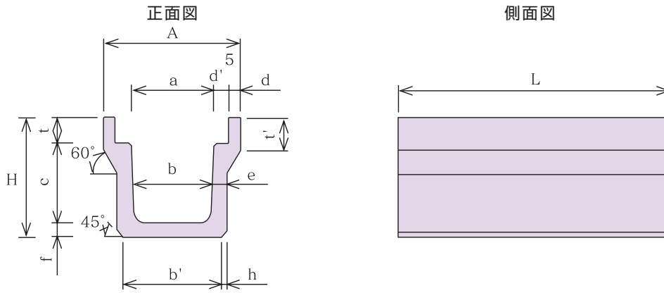
寸法表 (車道用)
