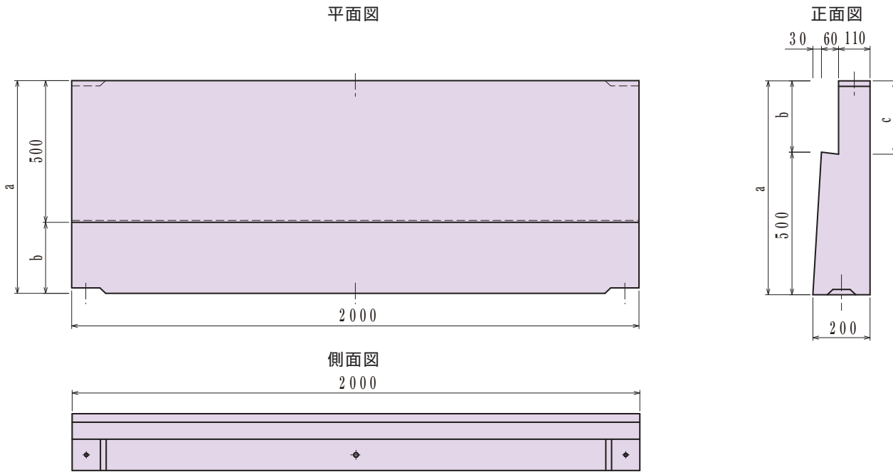
寸法表
