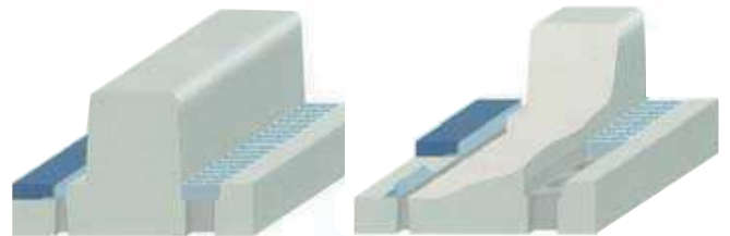
[3] 緑石付き両面取水型 歩道側は15mm幅のスリット、車道側は60mmのグレーチング構造です。 一つの側溝で歩道と車道の両側から取水できます。
