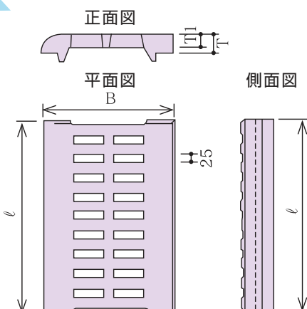
寸法表
