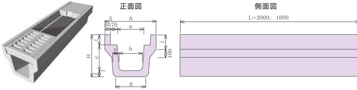
寸法表 単位(mm)
