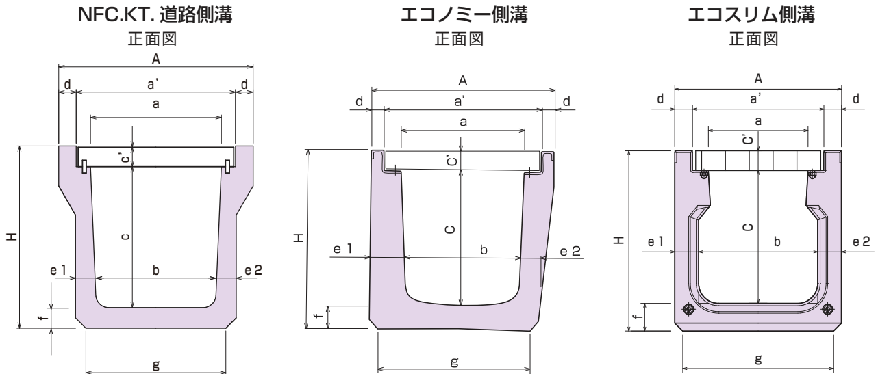
寸法表
